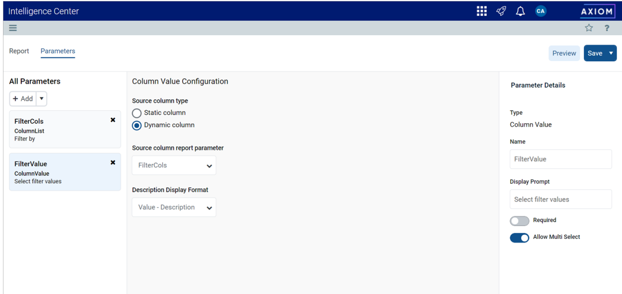
Example Column Value parameter using a Column List parameter to provide the source column
